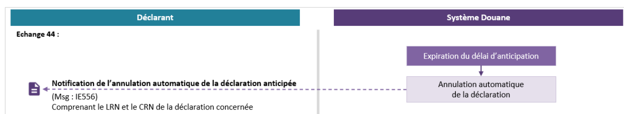
Figure 21 : Processus d'annulation automatique d'une déclaration d'exportation anticipée
