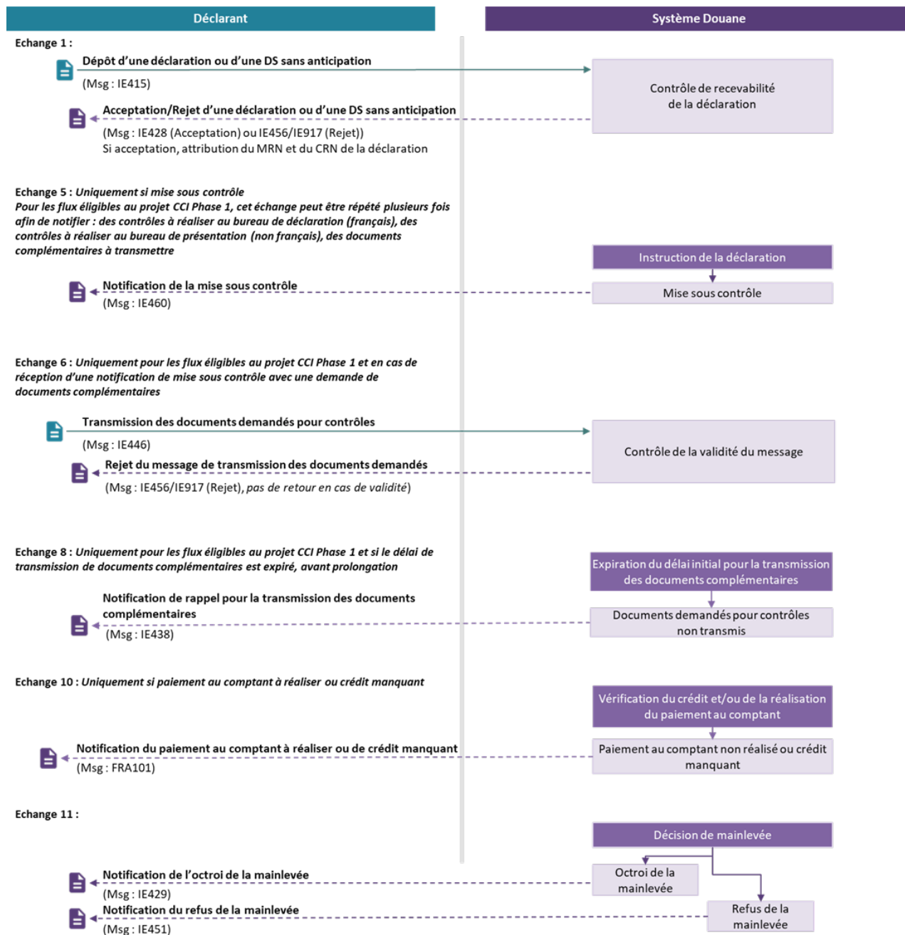
Figure 1 : Dédouanement à l'importation avec une déclaration sans anticipation
