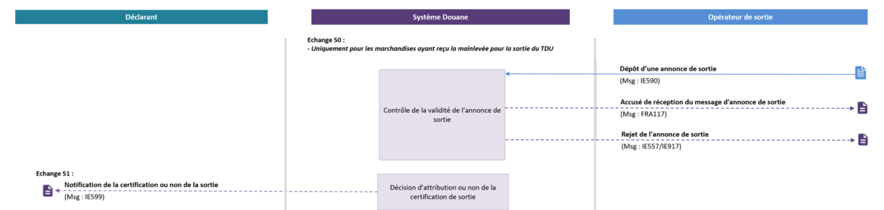
Figure 28 : Processus de sortie immédiate (sans stockage) de marchandises lorsque le bureau de sortie est confondu avec le bureau d'exportation
