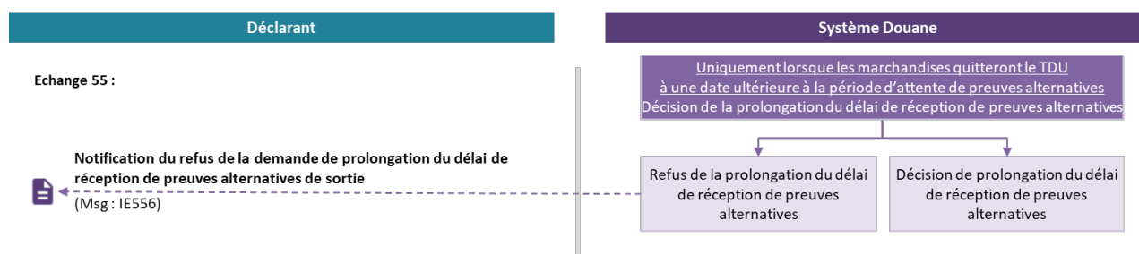
Figure 94 : Diagramme de séquence Échange 55
