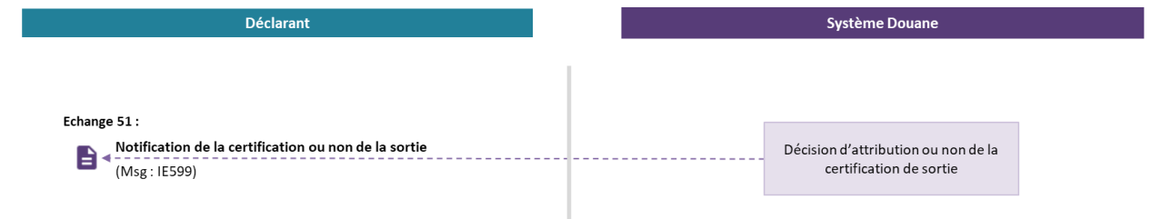
Figure 26 : Processus de sortie de marchandises sous transit au bureau d'exportation (lorsque le bureau d'exportation est compétent pour le lieu de prise en charge des marchandises)
